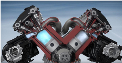
Zylinderabschaltung
