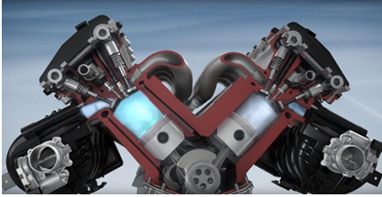
Zylinderabschaltung
