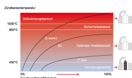
Zündkerzentemperatur
