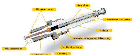
Querschnitt einer Zündkerze
