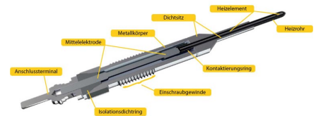
Querschnitt Keramikglühkerzen
